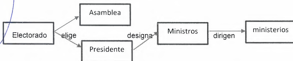
Gráfico 1: El modelo presidencialista
