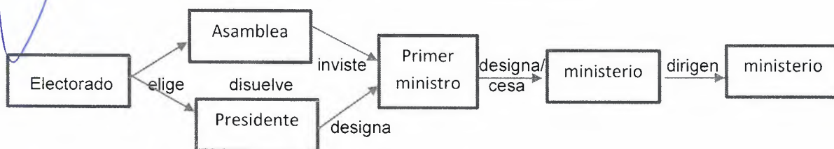
Gráfico 3: El modelo semipresidencialista
