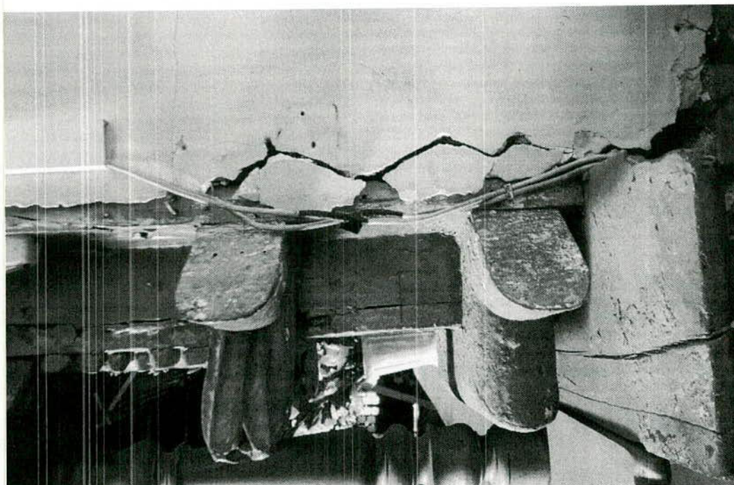
Estado de conservación general de la iglesia matriz
